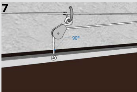
7 Plaats grote schroefhaak en bevestig katrol aan de schuif. Belangrijk: Touw moet loodrecht hangen!
