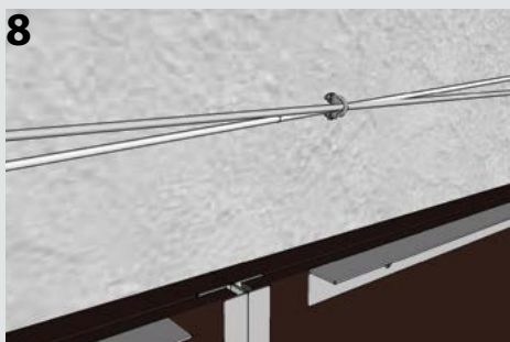
8 Bevestig het touwtje met een stalen kabelklem aan de staaldraad
